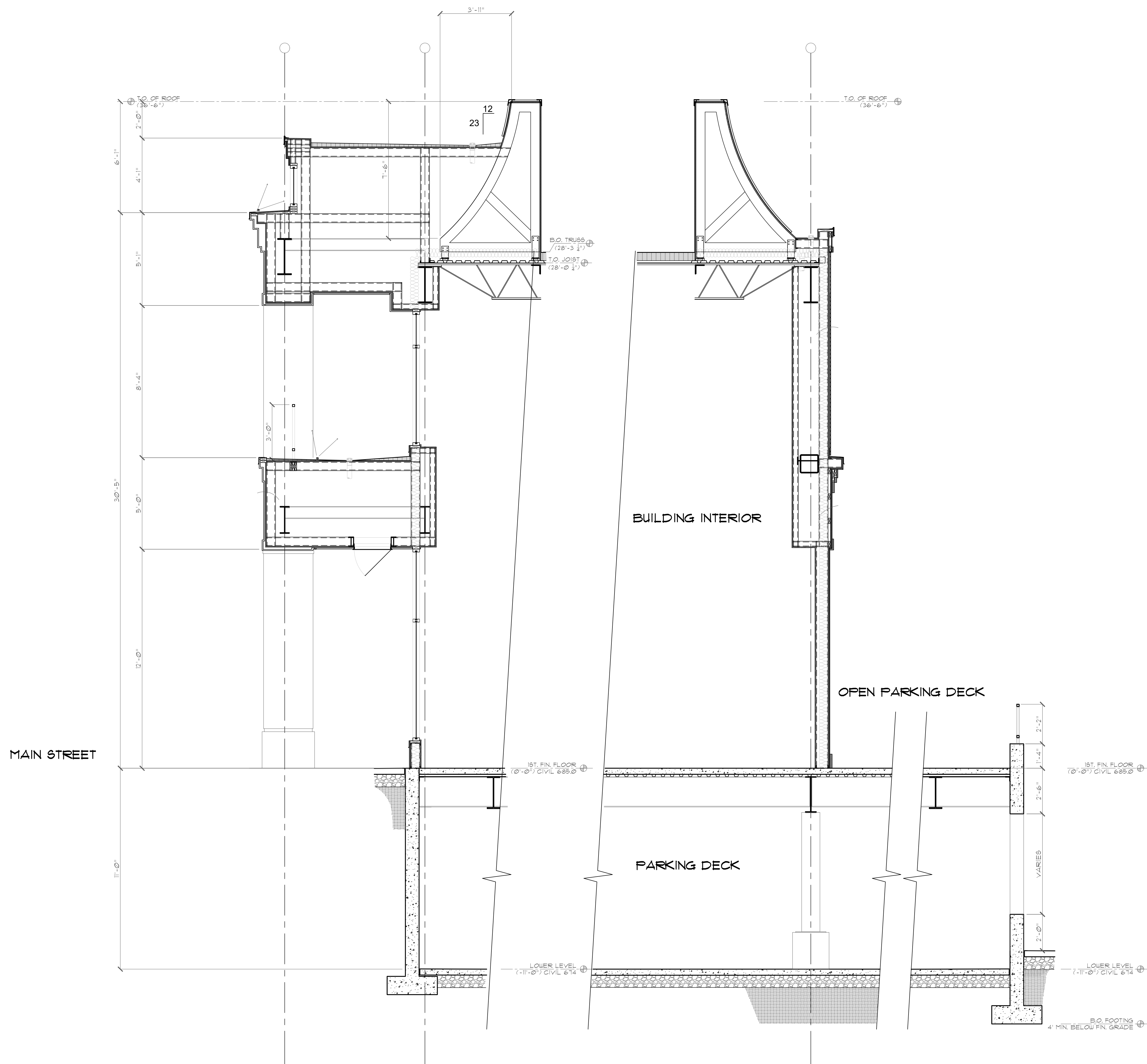
1 SECTION SCALE: 3/8"=1'-0"
